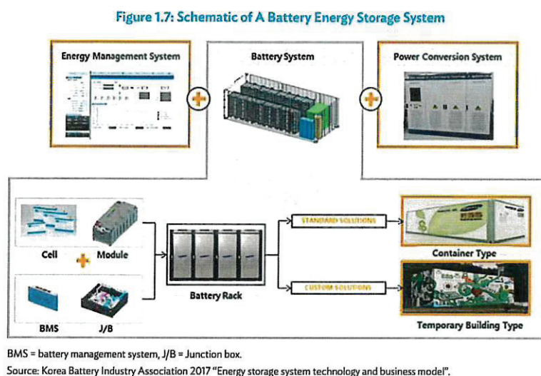
Figura 2 – Componenti di un BESS
